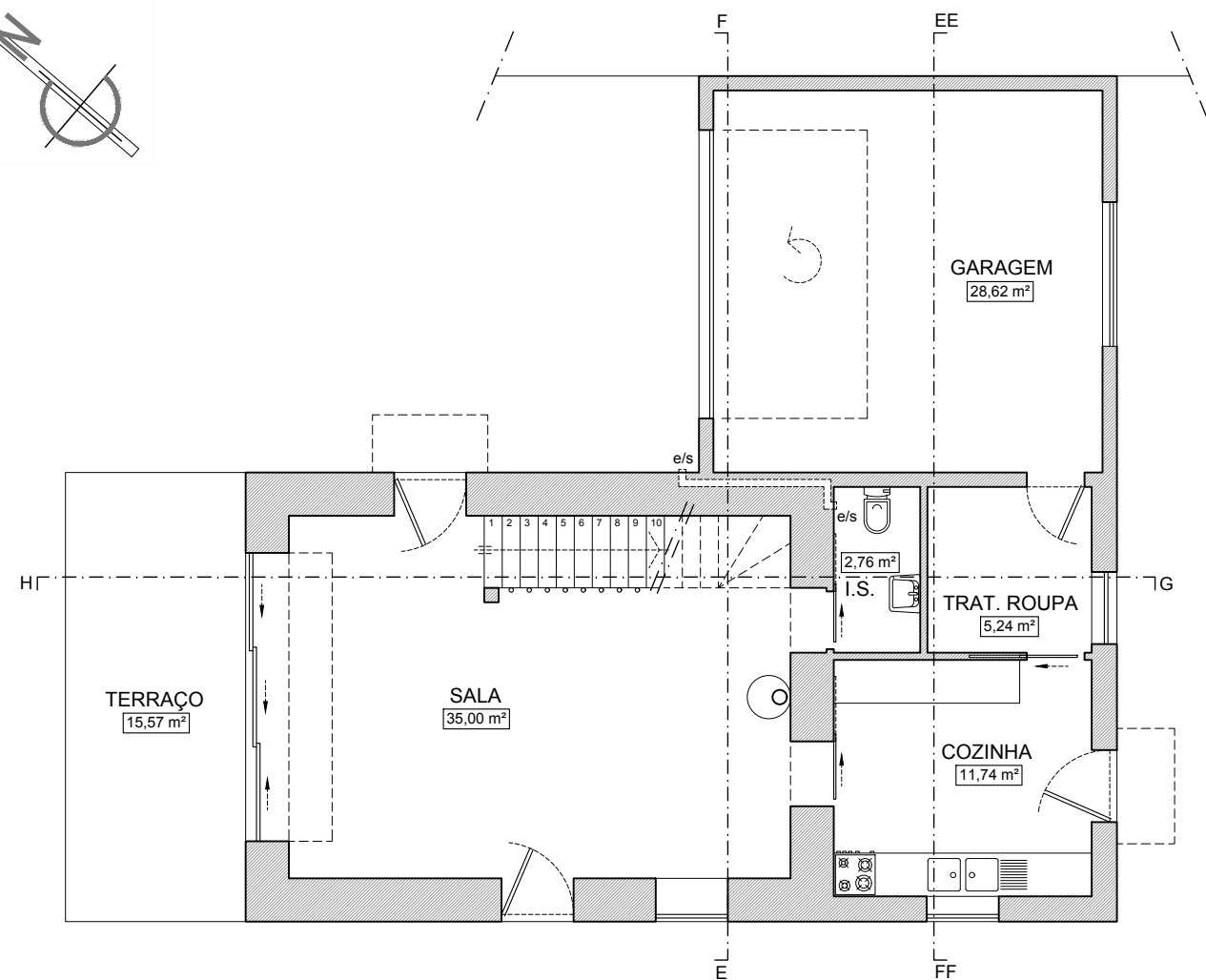
PI ANTA do RÉS-do-CHÃO
