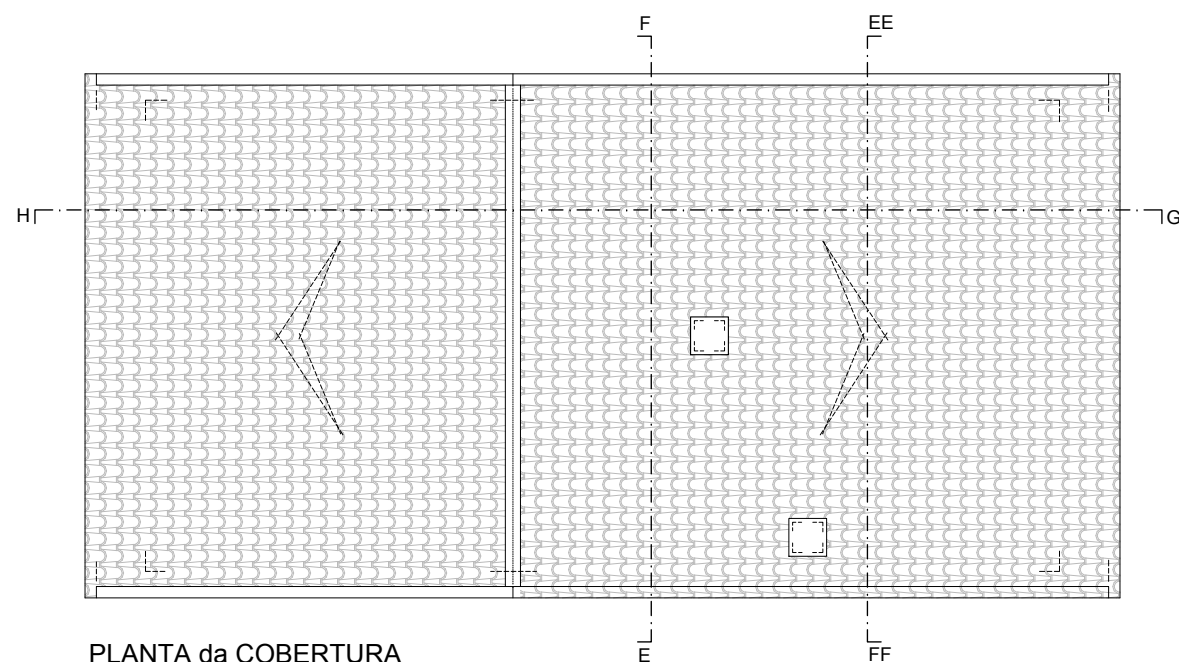
PLANTA da COBERTURA
