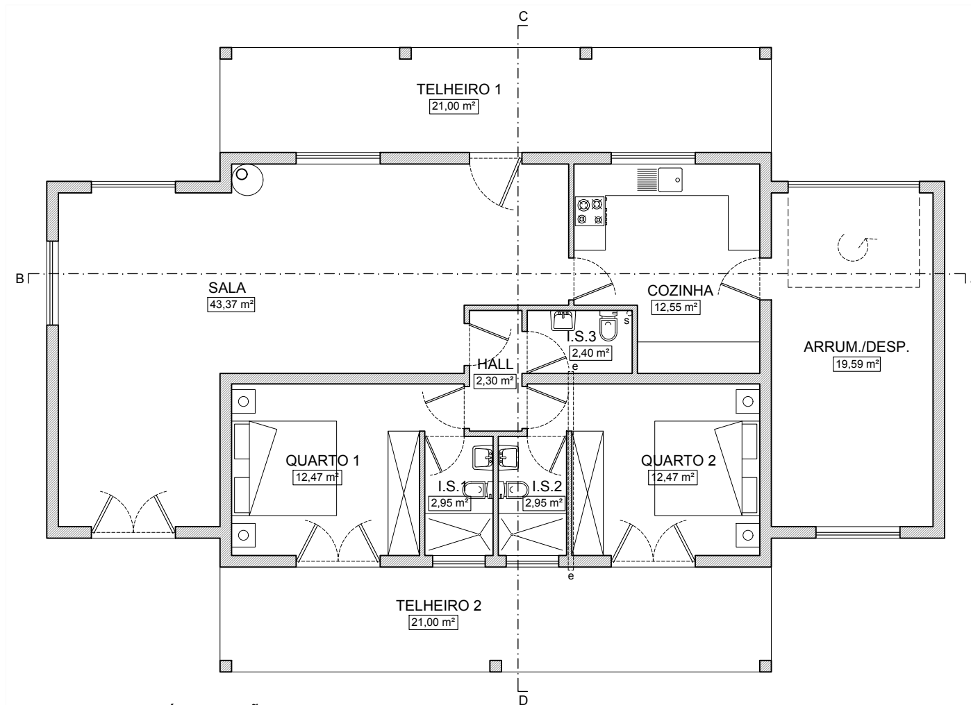
PLANTA do RÉS-do-CHÃO
