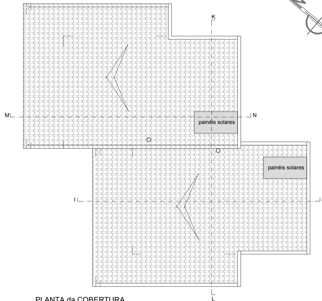
PLANTA da COBERTURA
